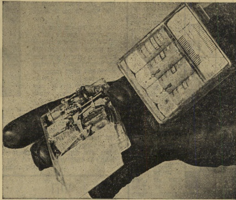
מכשיר יערי. בצילום: יד המחזיקה את שני חלקי המכשיר שנמצא צמוד למגירת שולחנו של מאיר יערי. החלק העליון מכיל סוללות, התחתון את משדר-הננס, ששידר לתחנת קליטה.
