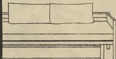
דגם 226 — טפה כפולה 190 x 57,6 x 70 ספה תחתית 70 x 25 x 190.
