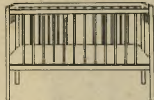
דגם 59A — מיטת תינוק בשני גדלים: 120x90x60, 140x90x60
