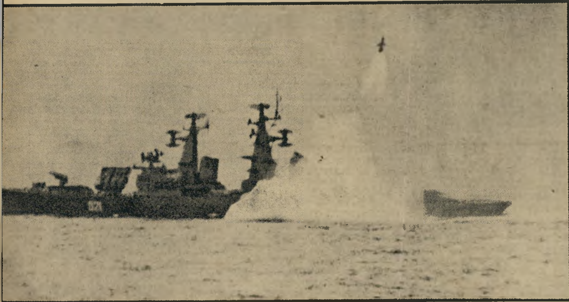
טיל נגד מטוסים נורה מעל סיפון אוניית מלחמה סובייטית מדגם קינדה, האוניות מדגם זה מצוידות במיתקני שיגור טילים מדגם גואה, שהוא הסאם-3. טילים אלה מגלים לפגוע במטוסים הססים במרחק של עד 30 ק"מ מכך שיגור, אולם מיומנותם עדיין לא הוכחה במיבצעים קרביים ממ
