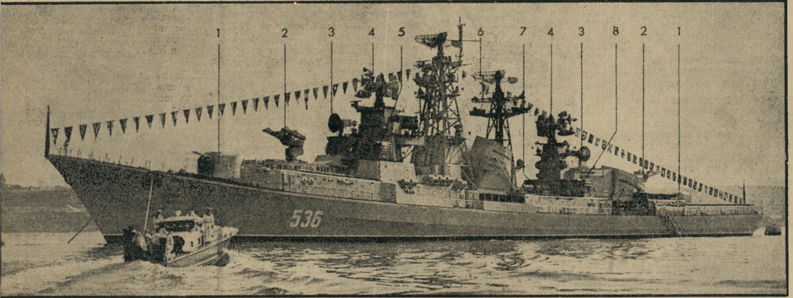
משחתת סובייטית חמושת-טילים זות בצי היס התיכון הסובייטי, מיועדת בעיקר ללחימה נגד מטוסים ונגד צוללות. היא חמושה בשני מיתקני שיגור טילים סאם-3. המספרים מציינים את מערכות הנשק שלה: (1) מדגם קאשיין, כמוה מצוידות אוניות אחר-זות בצי היס התיכון הסובייטי, מיועדת בעיקר ללחימה נגד מטוסים ונגד צוללות. היא חמושה בשני מיתקני שיגור טילים סאם-3. המספרים מציינים את מערכות הנשק שלה: (1)
