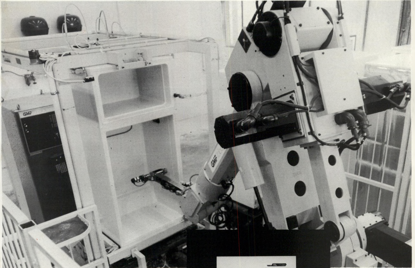
בתמונה: אחד הרובוטים המתוכננים של אמקור בפס הייצור של מקררי אמקור XL עובד. שעות נוספות.
