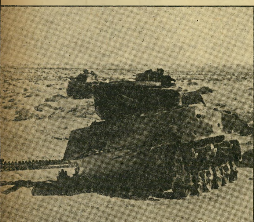
טאנק ישראלי מדגם שרמן מוסל בצד הכביש. הסימנים מעידים כיצד חוסל הוא וחבריו: מוקש קרע את השרשרת, ופגזים חודרי-שריון נקבו את דפנותיו המוננים פחות.
