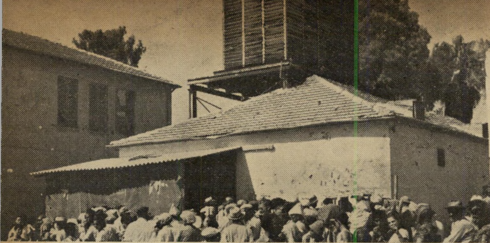
מגדרי הקירור : סימן ההיכר של "מכרה הקרח" : לפני הכנסתם לתבניות הקרח מועברים דרכו המים, כדי לקררם בכמה מעלות — דבר המקל על הקפאתם. בחו"ל גדולה התפוקה של אותן מכונות, בגלל האקלים הקר והימצאות צינורות המים בעומק רב יותר באדמה. נארץ אטי התהליך ככל שנדל החום.
